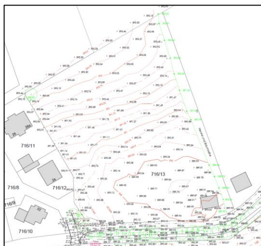
Abb. 9 Planausschnitt Vermessung; Quelle Plan: MAK Vermessung GbR, 21.01.2020
